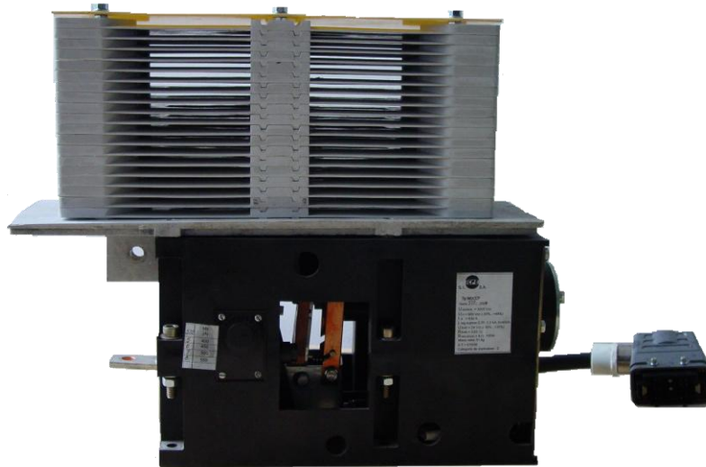
Întreruptor monopolar 800V /630A c.c
